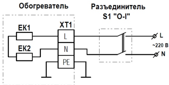
Рис. 2.2 Схема подключения обогревателя НС-2.0
